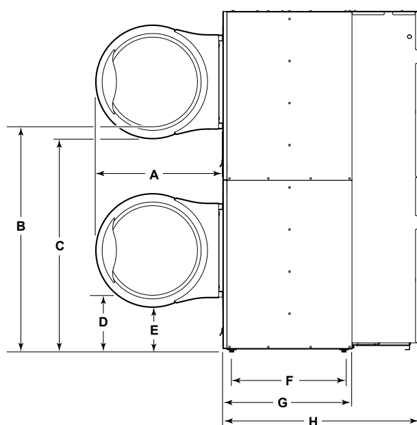
Côté droit
